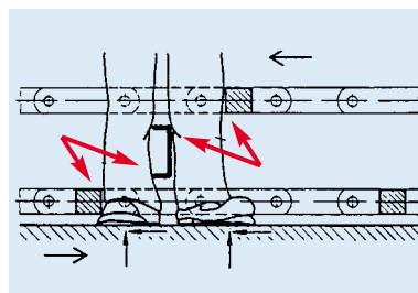
Abb. 31: Gefahrstelle zwischen den umlaufenden Ketten
