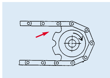
Abb. 29: Gefahrstelle an einem Kettenumlenktrah
