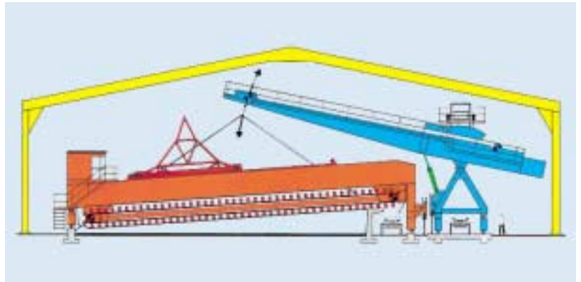
Abb. 1: Fahrbare Traggerüste
