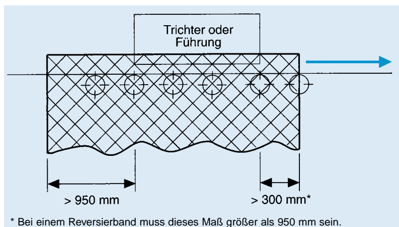
Abb. 11: Verdeckung eines Tragrollensatzes (Prinzipiskizze)
