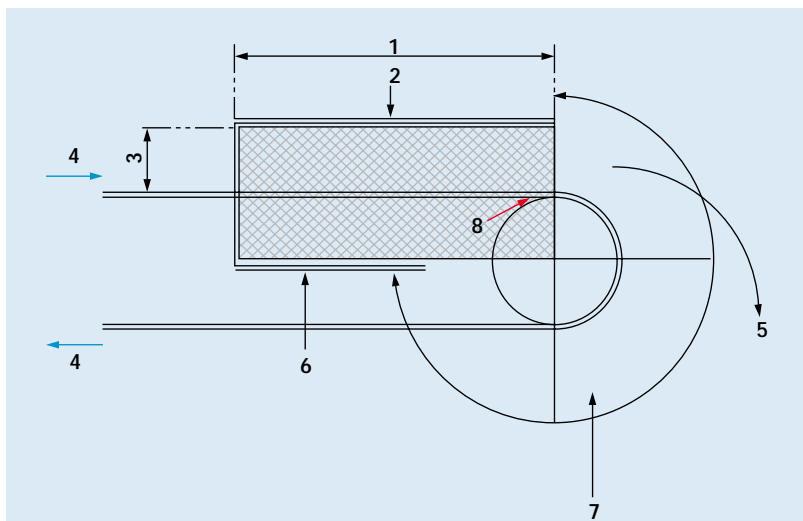
Abb. 4: Prinzip des Sicherheitsschutzes durch eine feststehende trennende Schutz-einrichtung an der Kopftrummel
