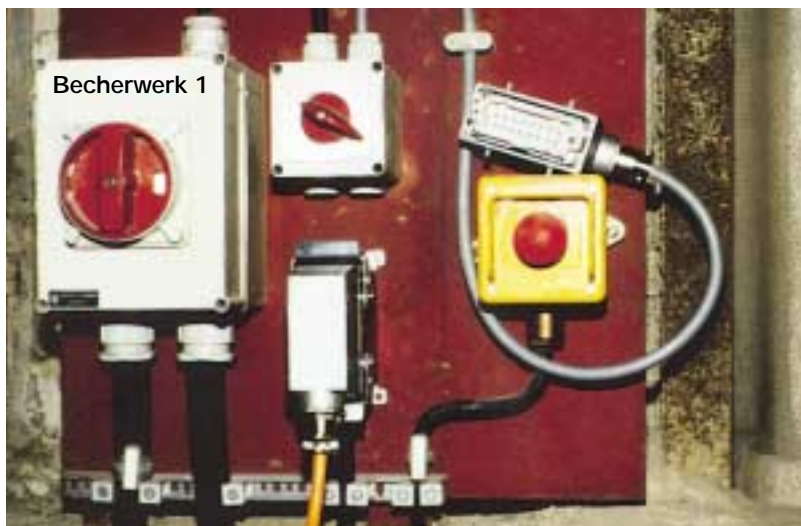
Abb. 40: Vor-Ort-Schalteinrichtung an einem Becherwerk
