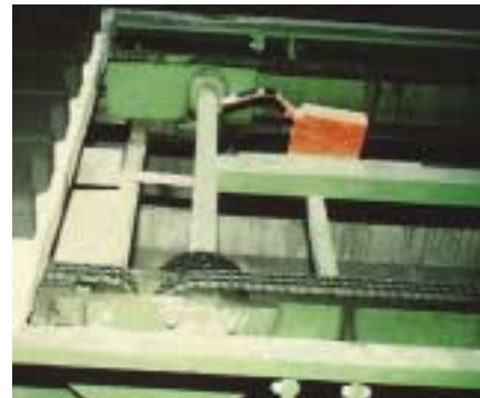
Abb. 35: Allseitige Verdeckung von Transportketten
